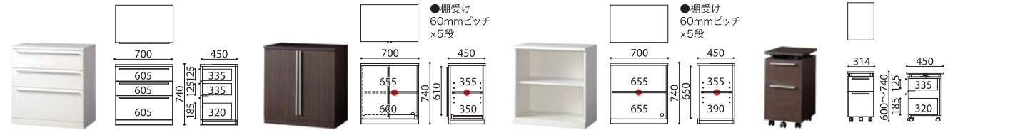
C1D-チェスト ホワイト No.6110130 C1D-チェスト ウェンジ No.6150136 ¥76,000(税抜) W700xD450xH740 重量31kg/1個口
