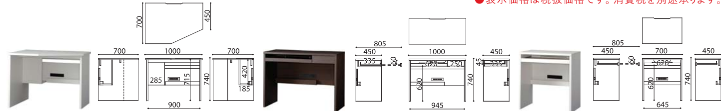
C1D-コーナーデスク左 ホワイト No.6110109 C1D-コーナーデスク左 ウェンジ No.6150105 ¥63,000(税抜) W1000xD700xH740 重量27kg/1個口
