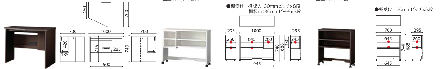
C1D-コーナーデスク右 ホワイト No.6110116 C1D-コーナーデスク右 ウェンジ No.6150112 ¥63,000(税抜) W1000xD700xH740 重量27kg/1個口
